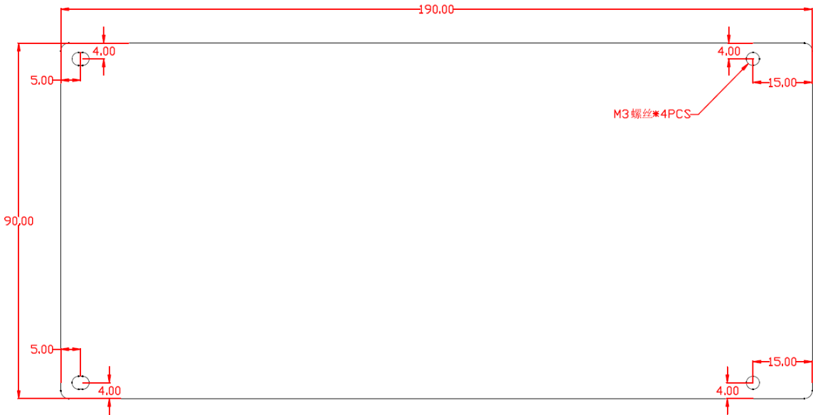
结构尺寸图（单位：毫米） Figure of structure size (Unit: mm)
